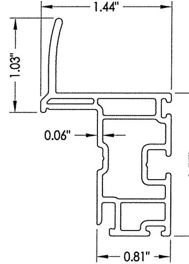
8 HANDLE STILE
